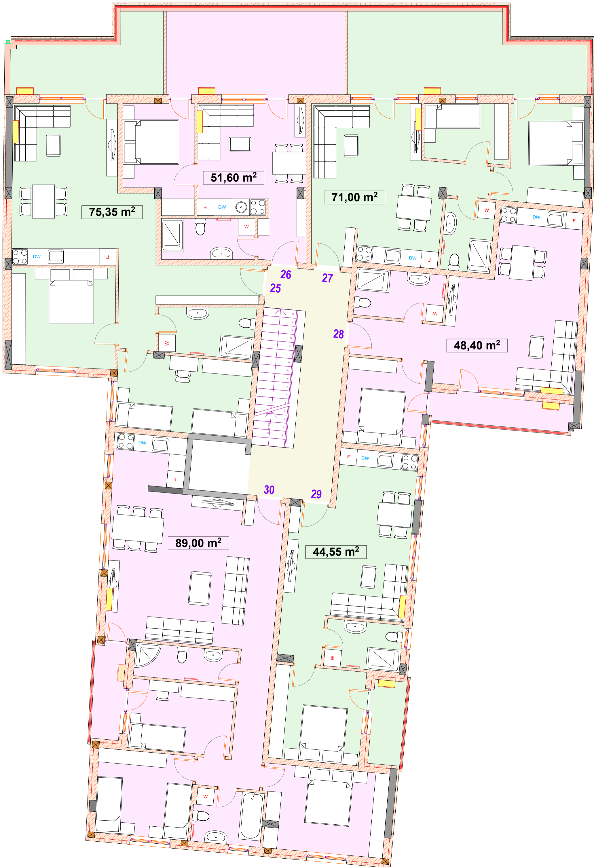
OSNOVA POVUČENOG SPRATA
