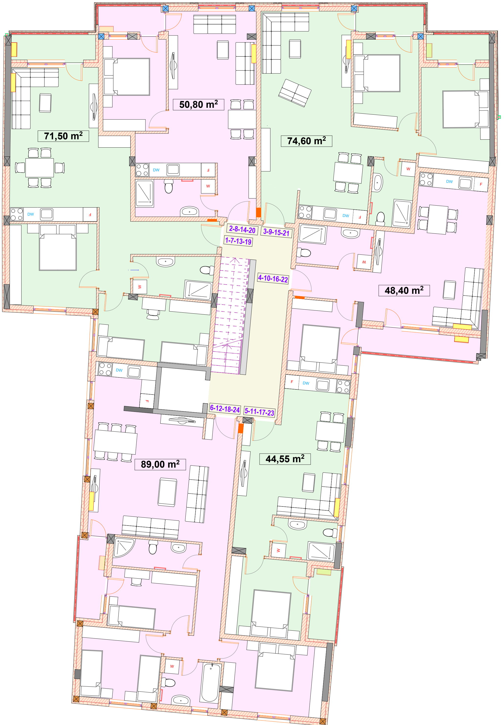
OSNOVA TIPSKOG 1-2-3-4 SPRATA
