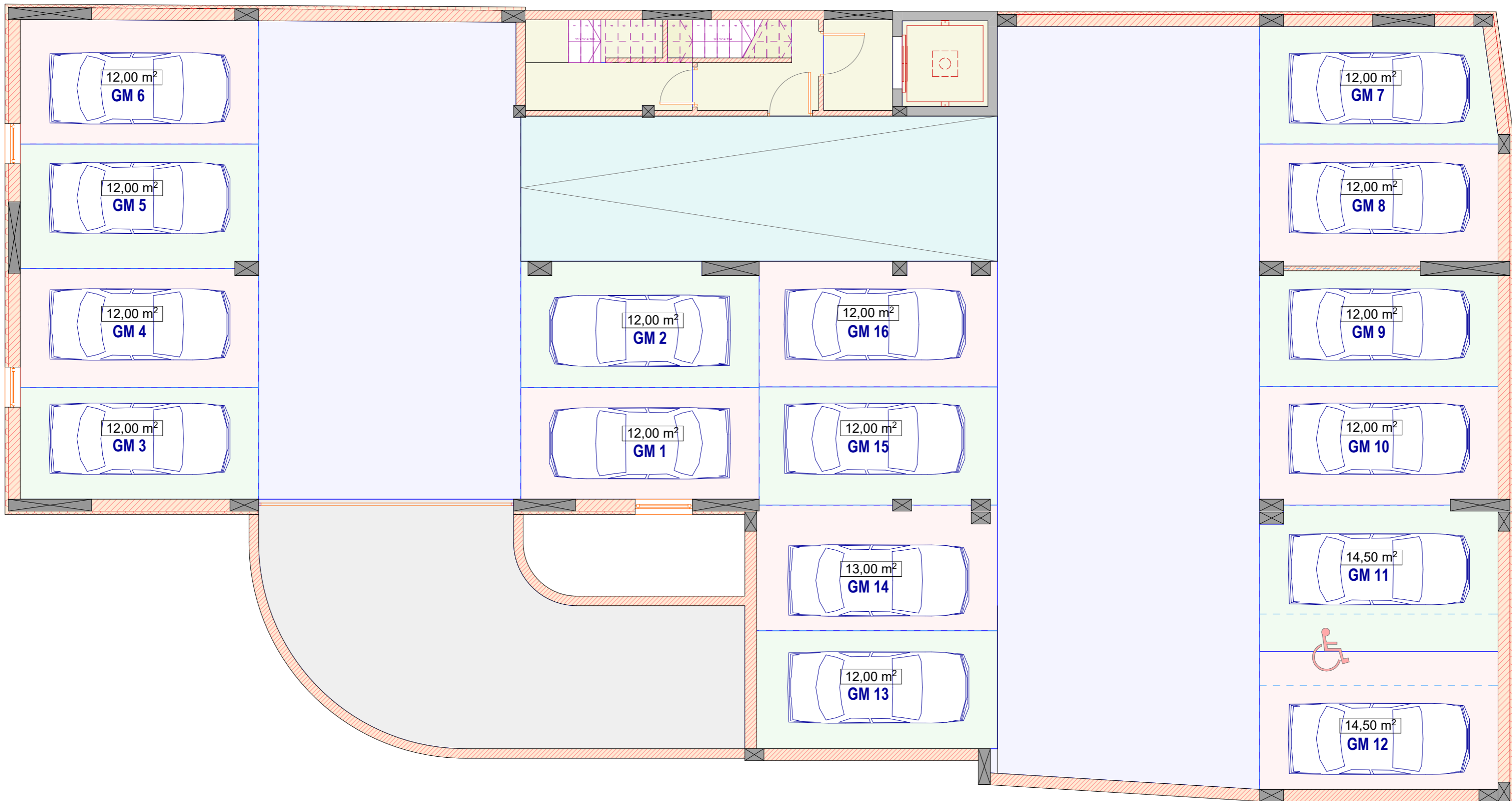
OSNOVA PODRUMA
